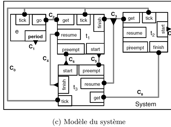
FIG. 3.16 – Modélisation d'un système multi-processeur avec BIP (source : [BBS06])
