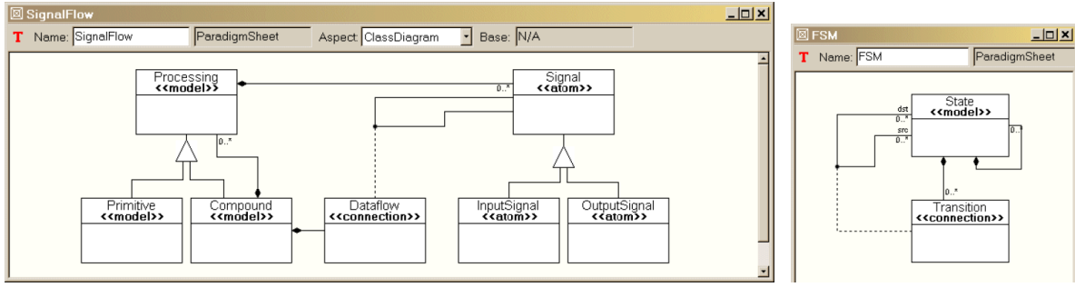
(a) Méta-modèle d'un langage à base de flots de données
